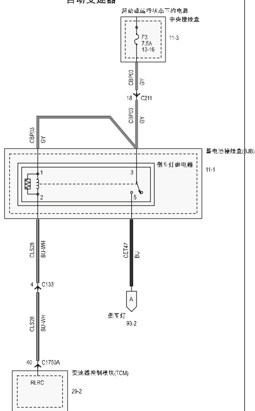
自动变速器
